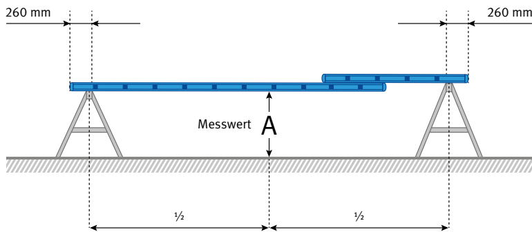
Abb. 16 Unbelastete Leiter
