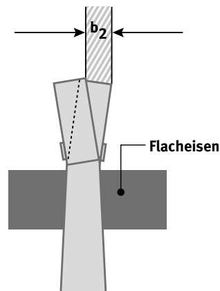
Abb. 21 Spiel der Spitzen senkrecht zur Bewegungs- bzw. Krafttrichtung
